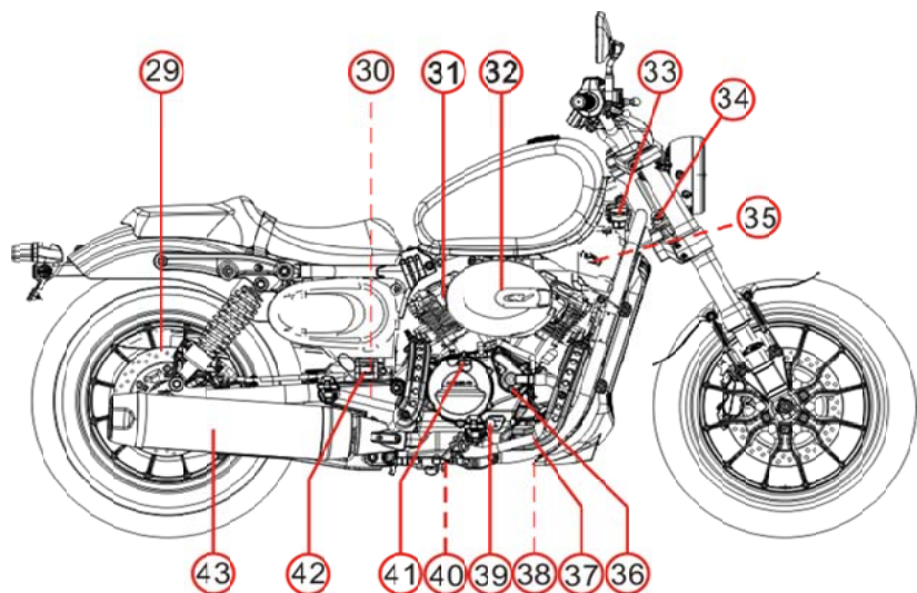
成车右侧图
