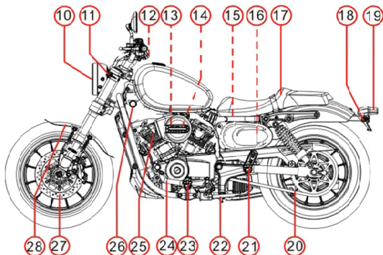
成车左侧图
