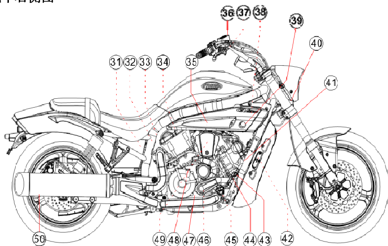
成车右侧图
