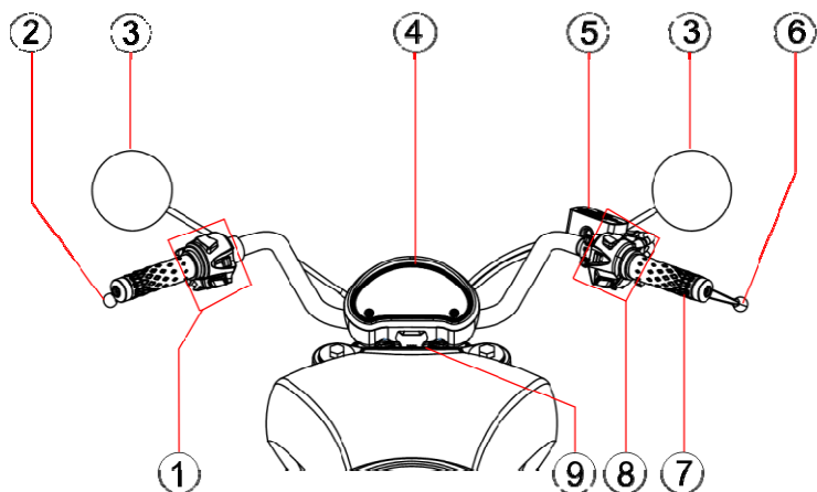
车把仪表
