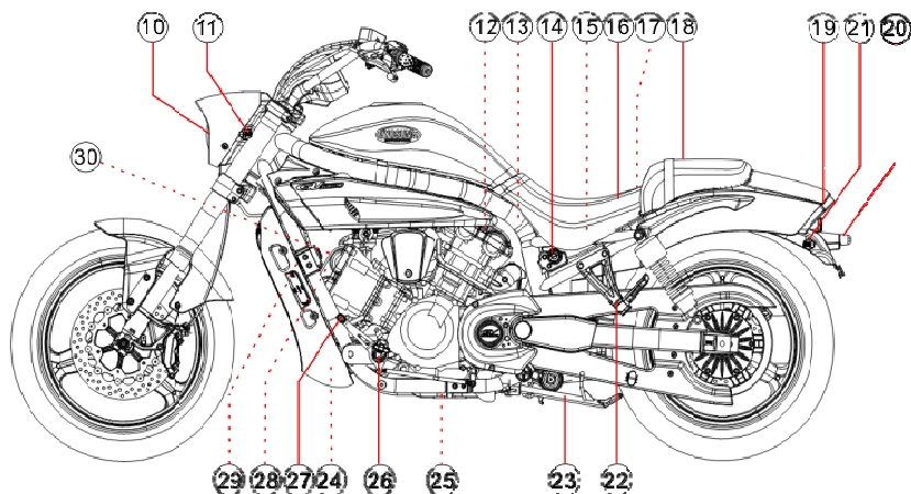
成车左侧图
