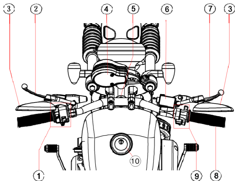
车把仪表
